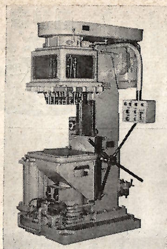
自動多軸孔明捻子立盤
